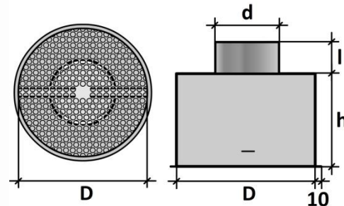
Obr.č. 6 ASK2 anemostatová krabica kruhová, prívodná s vrchným vývodom
