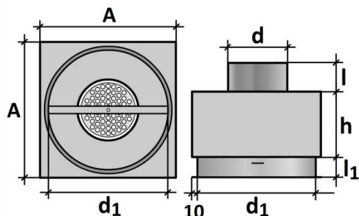
Obr.č. 3 ASHKV anemostatová krabica hranatá s kruhovými vývodmi- vrchný vývod
