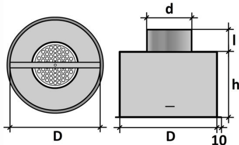
Obr.č. 5 ASK anemostatová krabica kruhová, odvodná s vrchným vývodom
