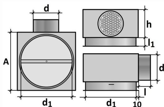
Obr.č. 1 ASHKB anemostatová krabica hranatá s kruhovými vývodmi- bočný vývod
