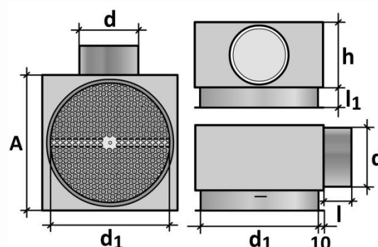
Obr.č.2 ASHKB2 anemostatová krabica hranatá s kruhovými vývodmi- bočný vývod
