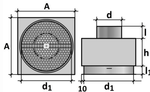
Obr.č. 4 ASHKV2 anemostatová krabica hranatá s kruhovými vývodmi- vrchný vývod
